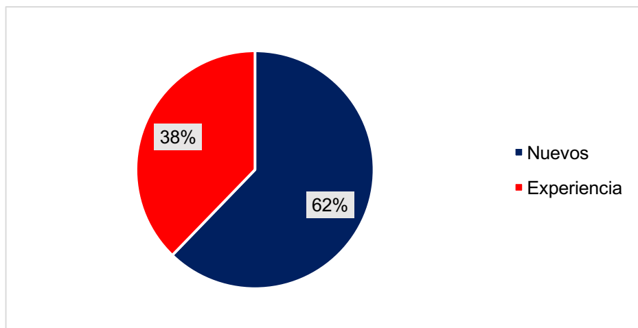
Gráfico 6: Candidatos Nuevos
