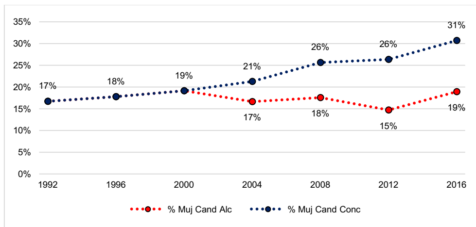
Gráfico 5: Mujeres Candidatas
