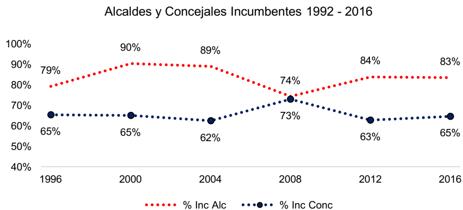
Gráfico 3: Incumbencia Municipal
